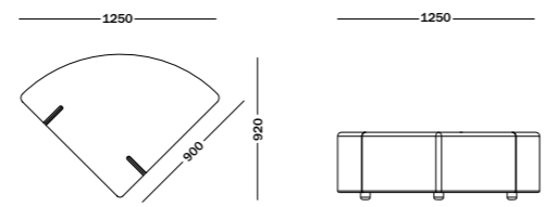
MODULE H - 90° angular module
