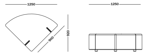
MODULE G - 90° angular module
